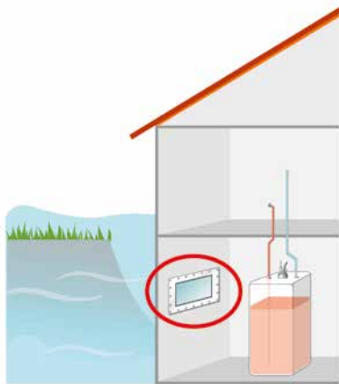
Variante 1: Aufstellraum gegen eindringendes Wasser sichern
